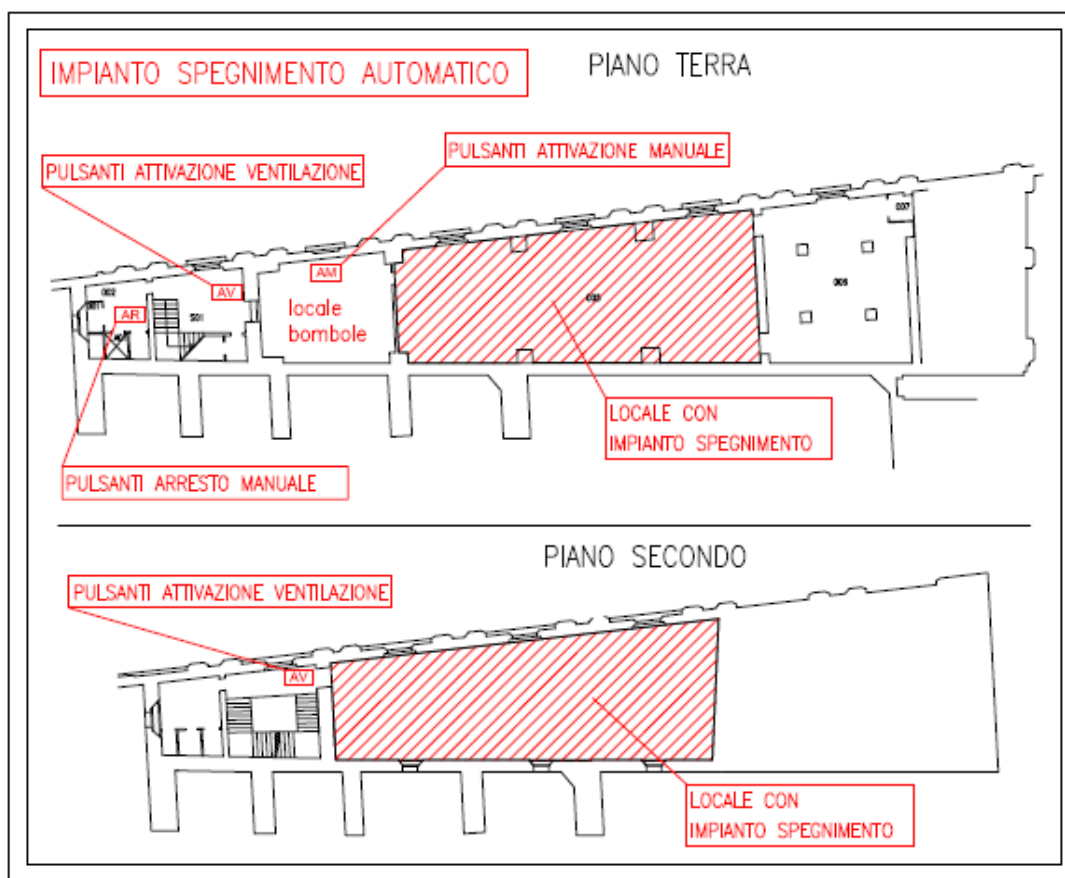
Figura 2 - Impianti spegnimento automatico.
