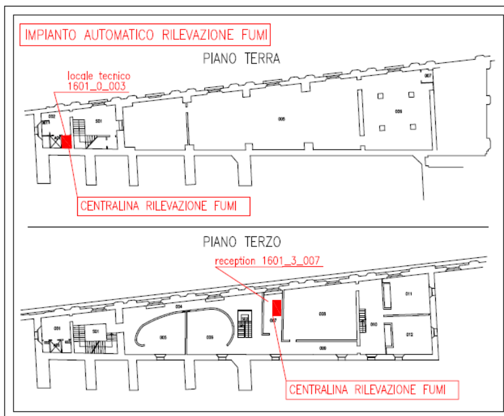
Figura 1. Impianti gestione emergenze.
