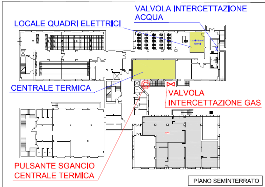
Figura 2.1 - Ubicazione impianti tecnologici – Piano Seminterrato.
