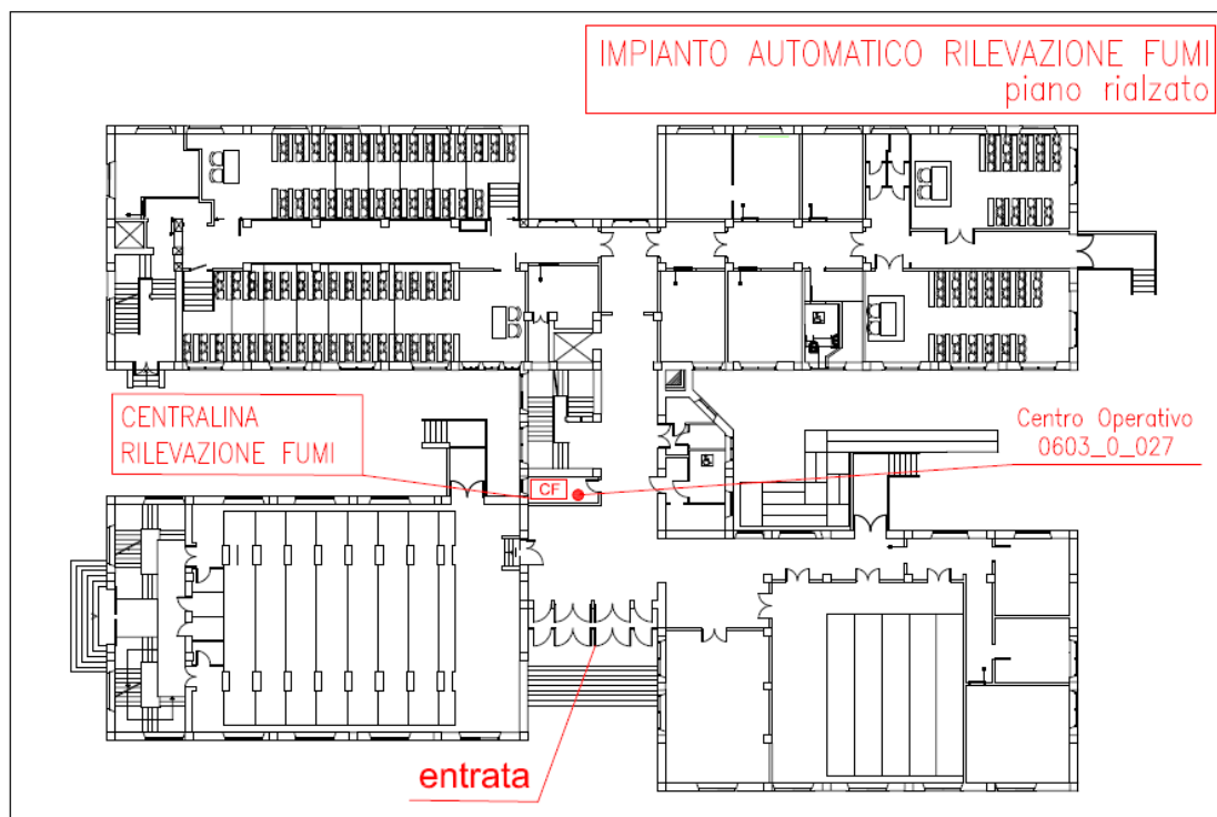
Figura 1. Impianti gestione emergenze.
