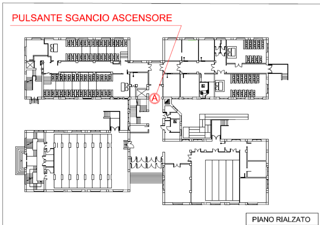
Figura 2.2 - Ubicazione impianti tecnologici – Piano Rialzato.
